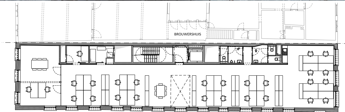
NIVEAU 1
